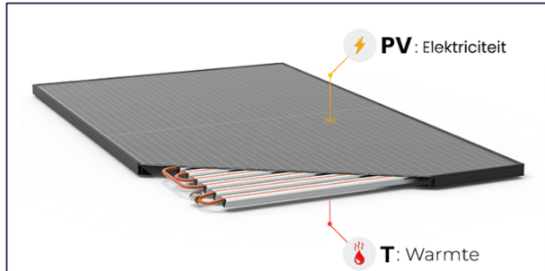
Figuur 3-4: Schematische weergave van een PVT-paneel
