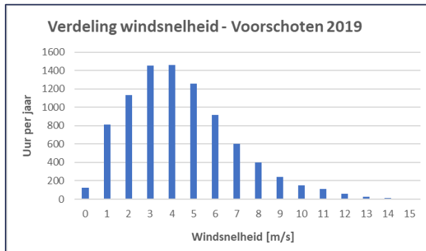
Figuur 3-9: Aantal uur dat gemeten windsnelheid per jaar voorkomt bij KNMI-meetlocatie Voorschoten
