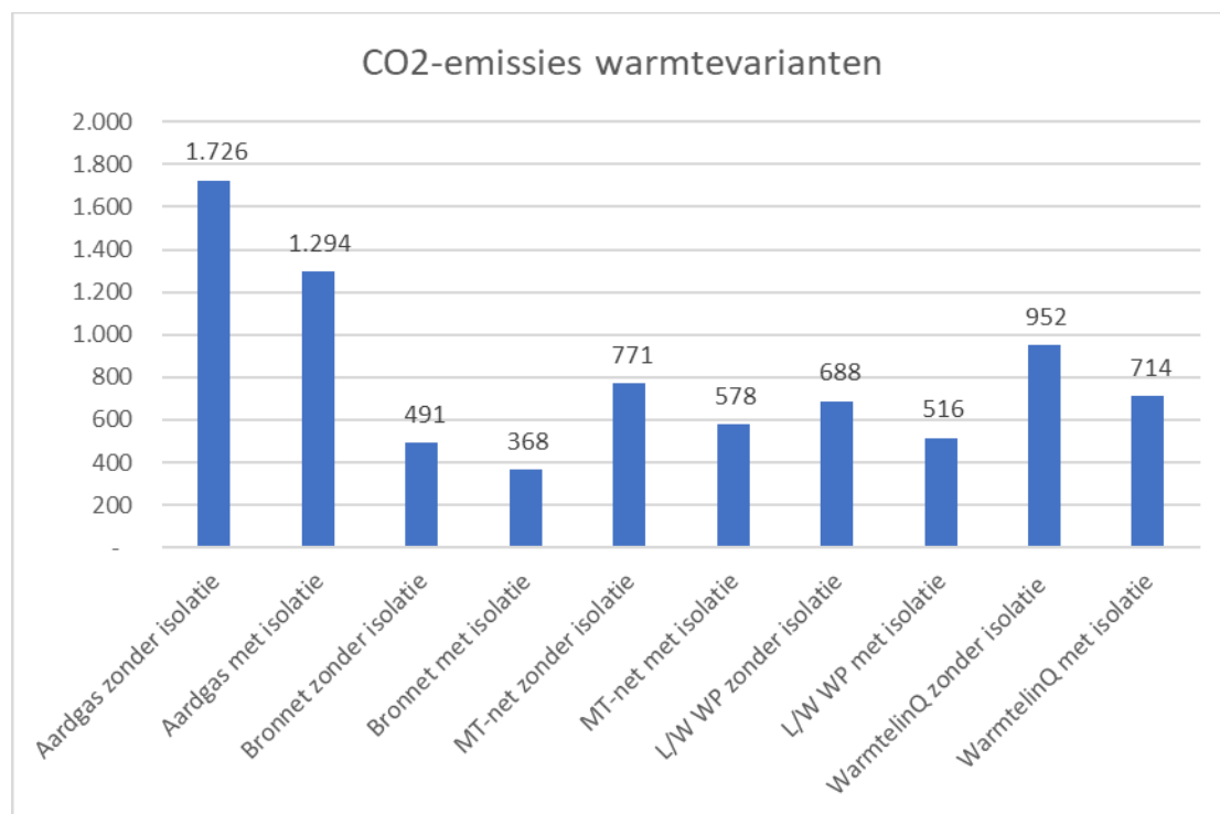
Figuur 7-2: Grafische weergave CO 2 -emissie warmtevarianten, in ton per jaar
