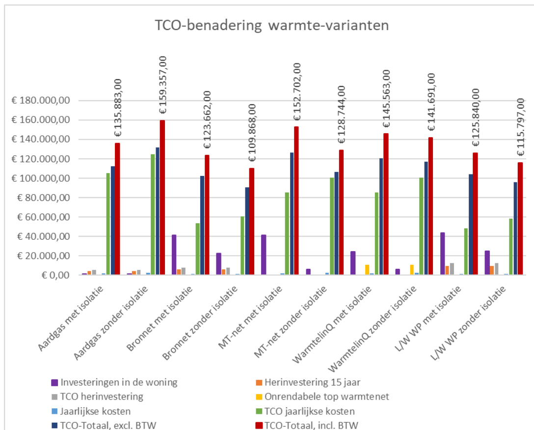
Figuur 1-3: Grafische weergave TCO-benadering doorerekende varianten. 'Zonder' betekent dat er geen aanvullende isolatiemaatregelen worden uitgevoerd. 'Met' betekent dat er wel isolatiemaatregelen zijn uitgevoerd. De ingeschatte kosten zijn in de berekeningen meegenomen.
