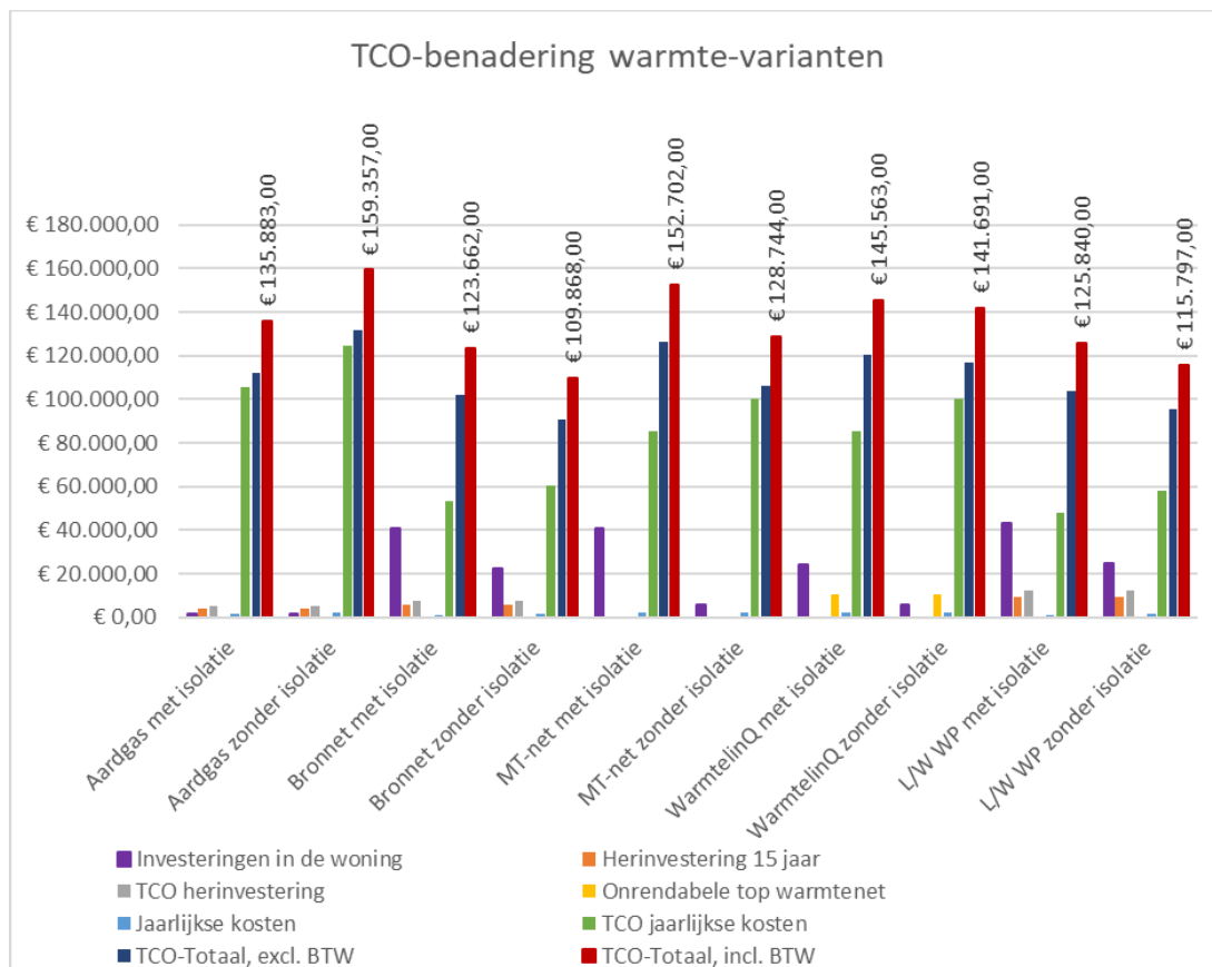
Figuur 7-1: Grafische weergave TCO-benadering doorgeredende varianten. 'Zonder' betekent dat er geen aanvullende isolatiemaatregelen worden uitgevoerd. 'Met' betekent dat er wel isolatiemaatregelen zijn uitgevoerd. De ingeschatte kosten zijn in de berekeningen meegenomen.
