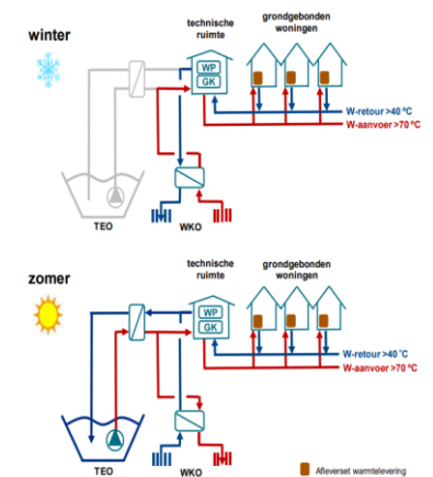
Figuur 3.12 | Principetekening concept 5. Een hoge temperatuur warmtenet en afleveraars in de woningen.
